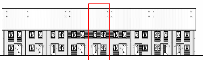
Voorgevel
