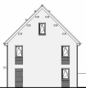
Rechter zijgevel
