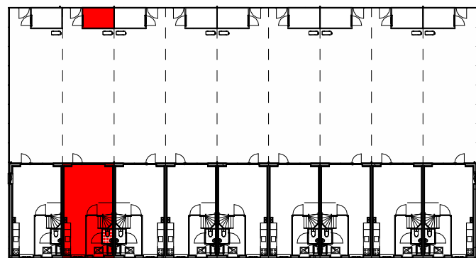
Begane grond
