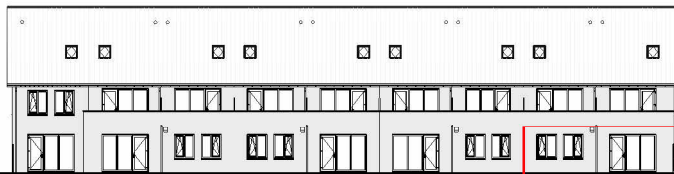
Achtergevel
