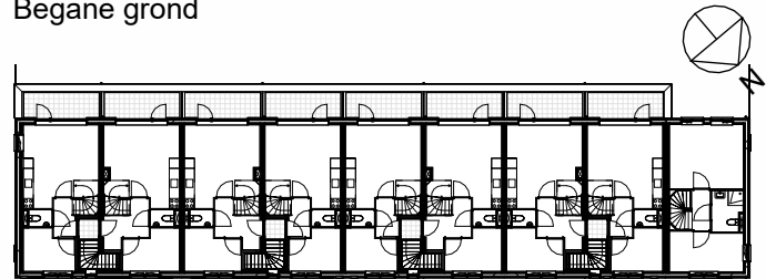
Begane grond
