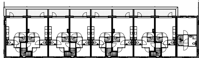
Eerste verdieping
