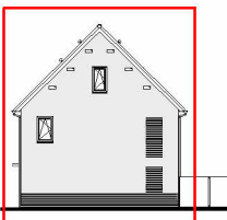
Rechter zijgevel
