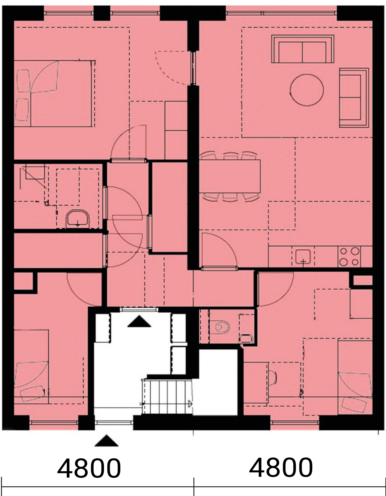
Begane grond
