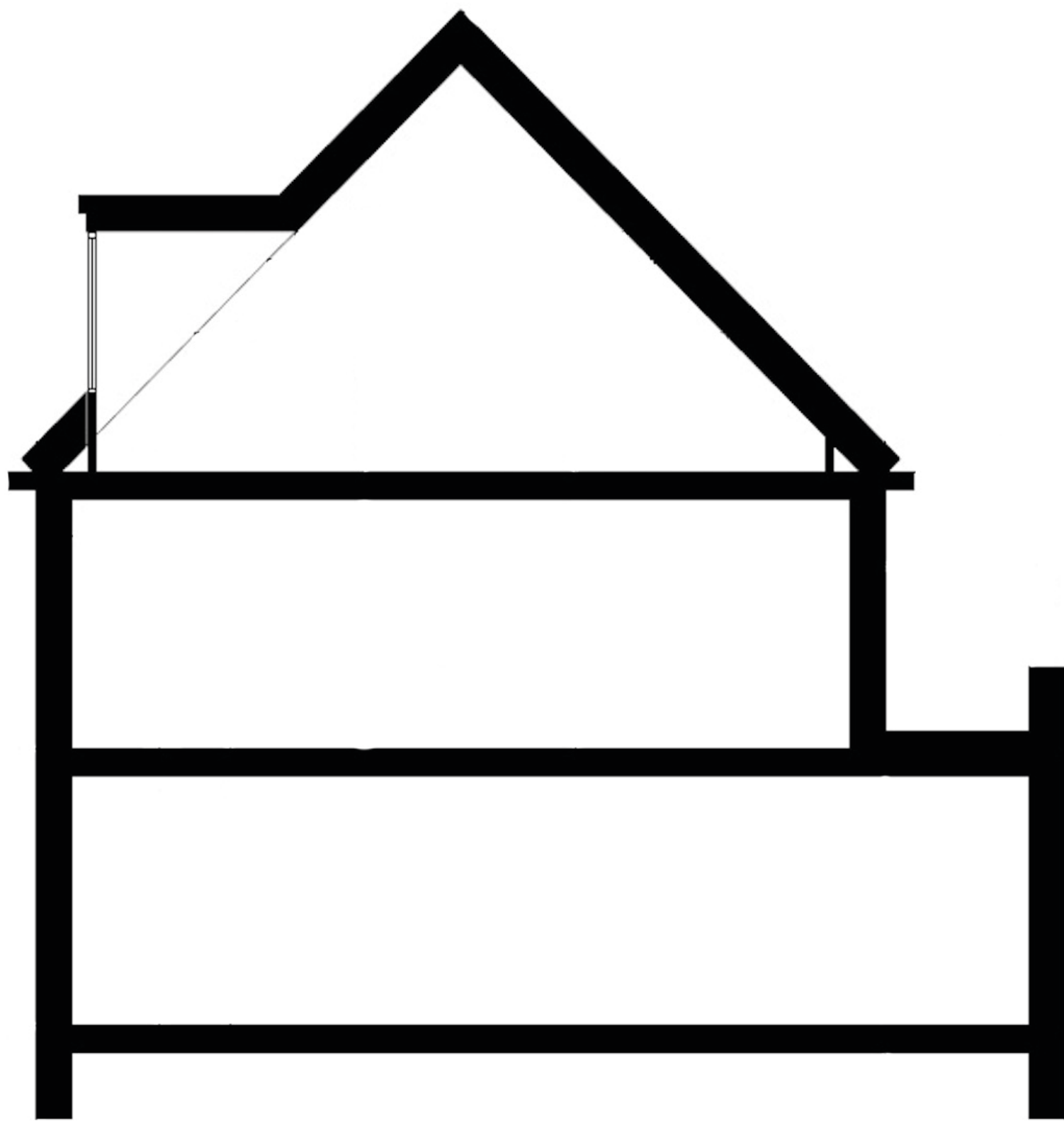
Dwarsdoorsnede
