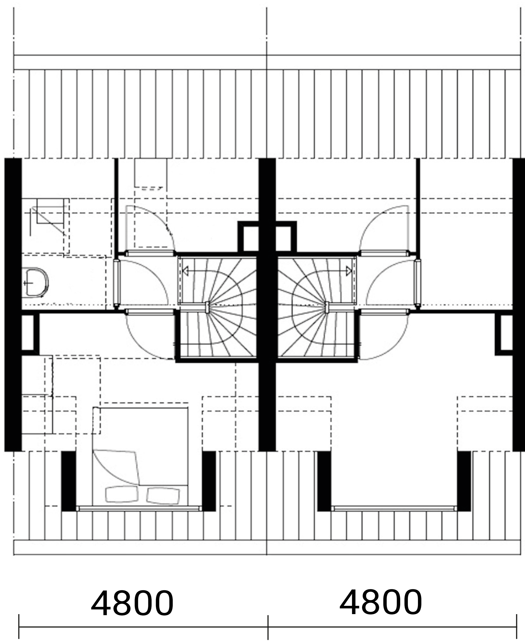
2e verdieping
