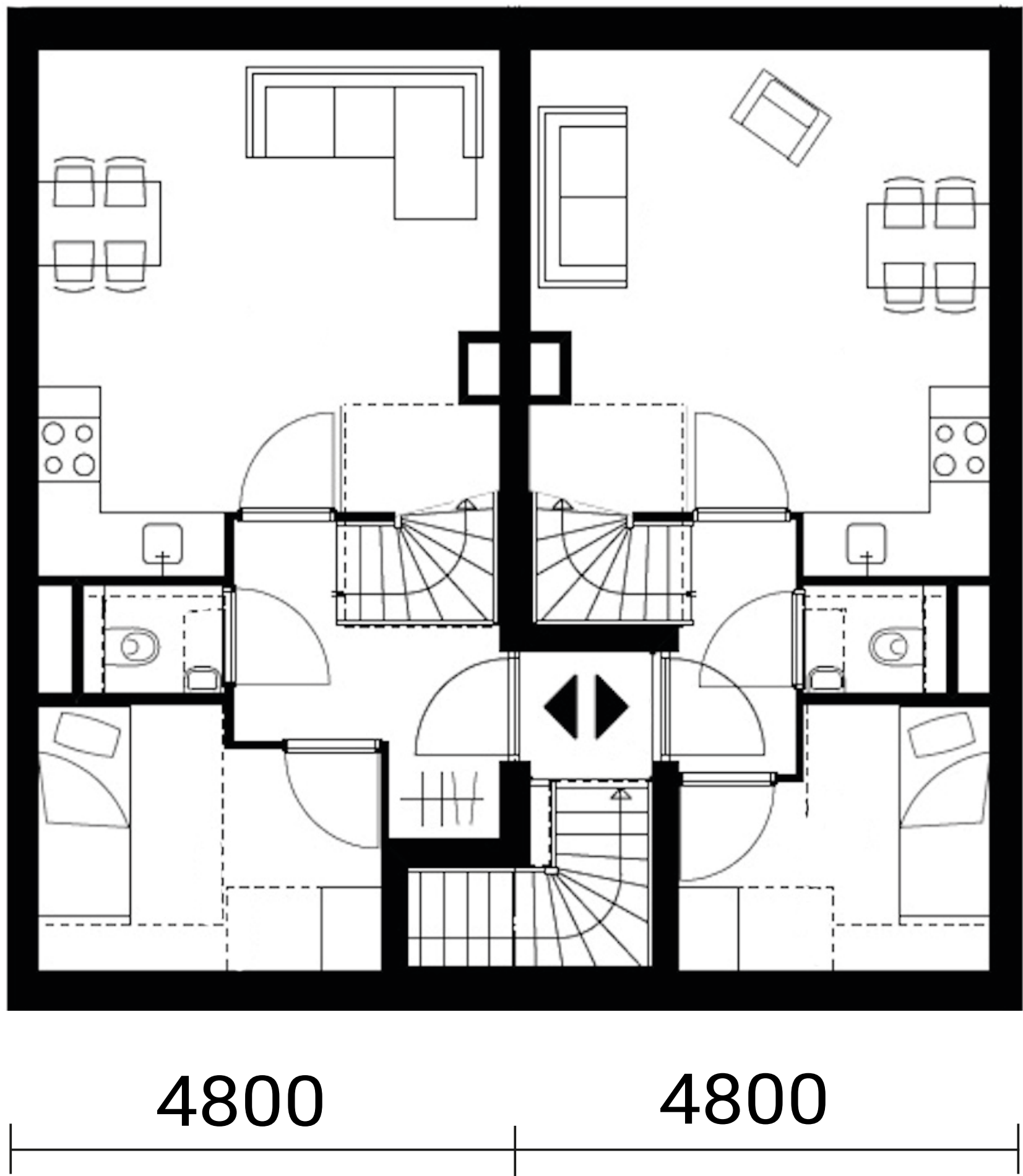
1e verdieping
